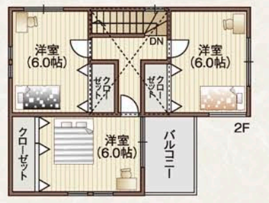
モデルハウス間取図
